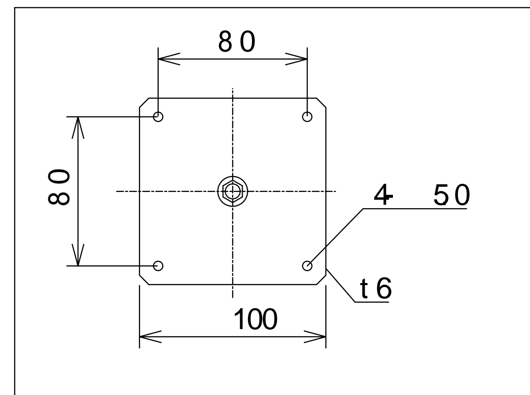
天井取付板寸法
