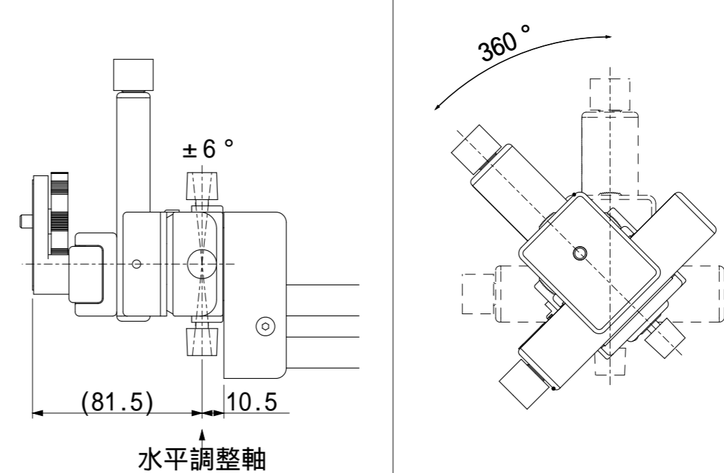
回転調整 (尺度2:1)
