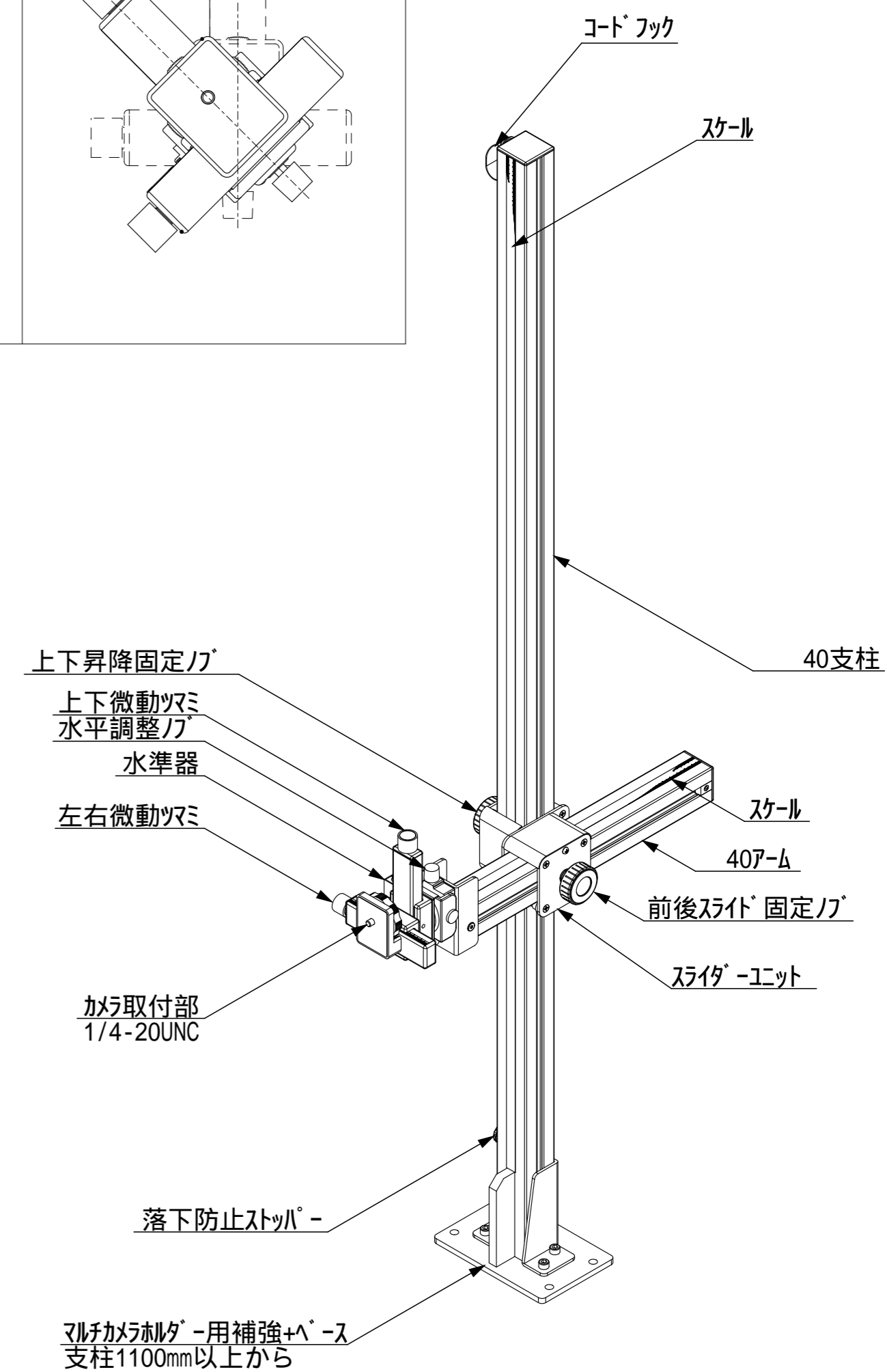
アーム各寸法
