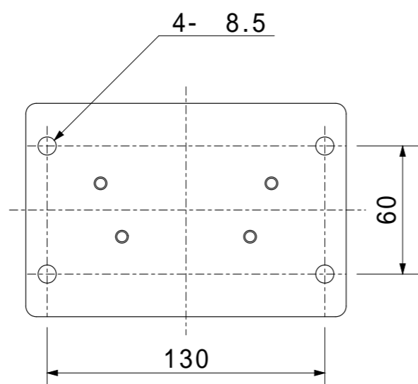
矢視A 取付面 (尺度2:1)
