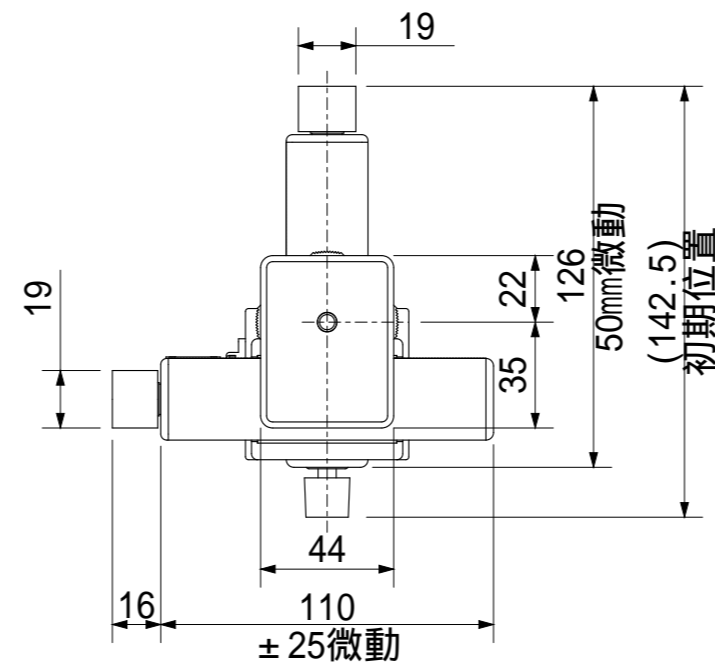
カメラ取付部 詳細 (尺度2:1)
