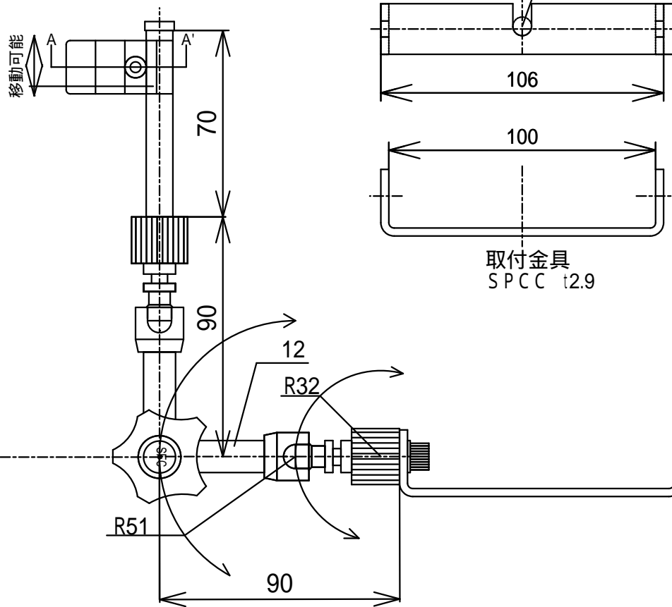
照明器ホルダーEX(シングル)
