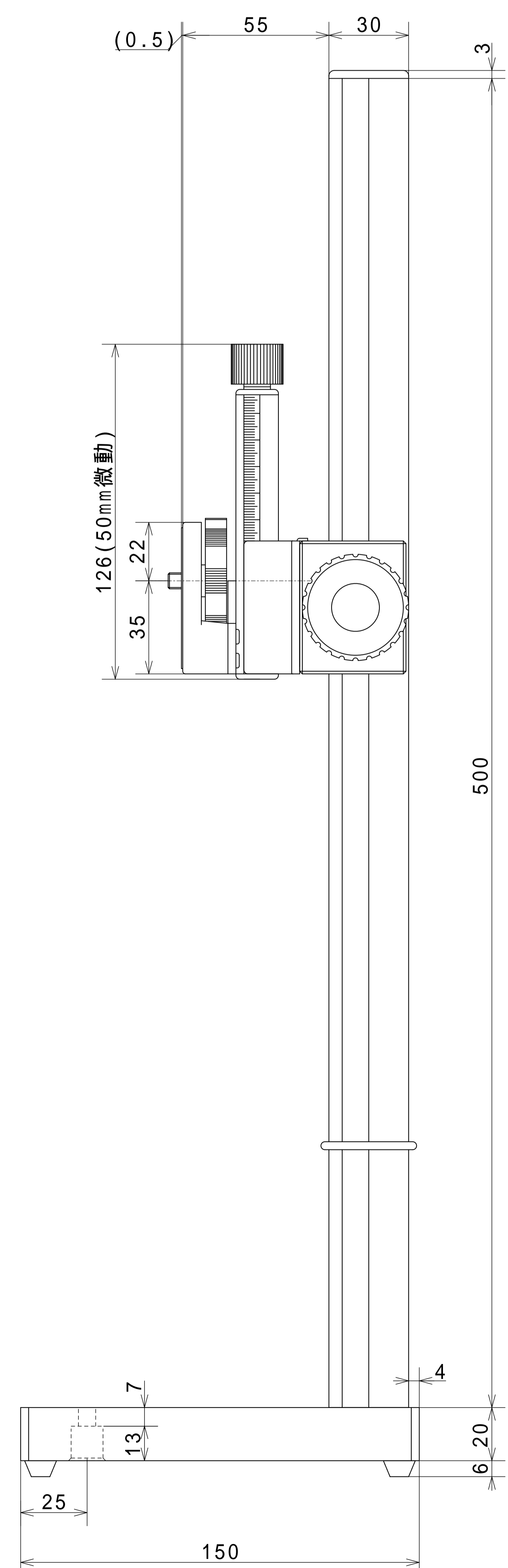
マイクロスタンド MK-2(500)
