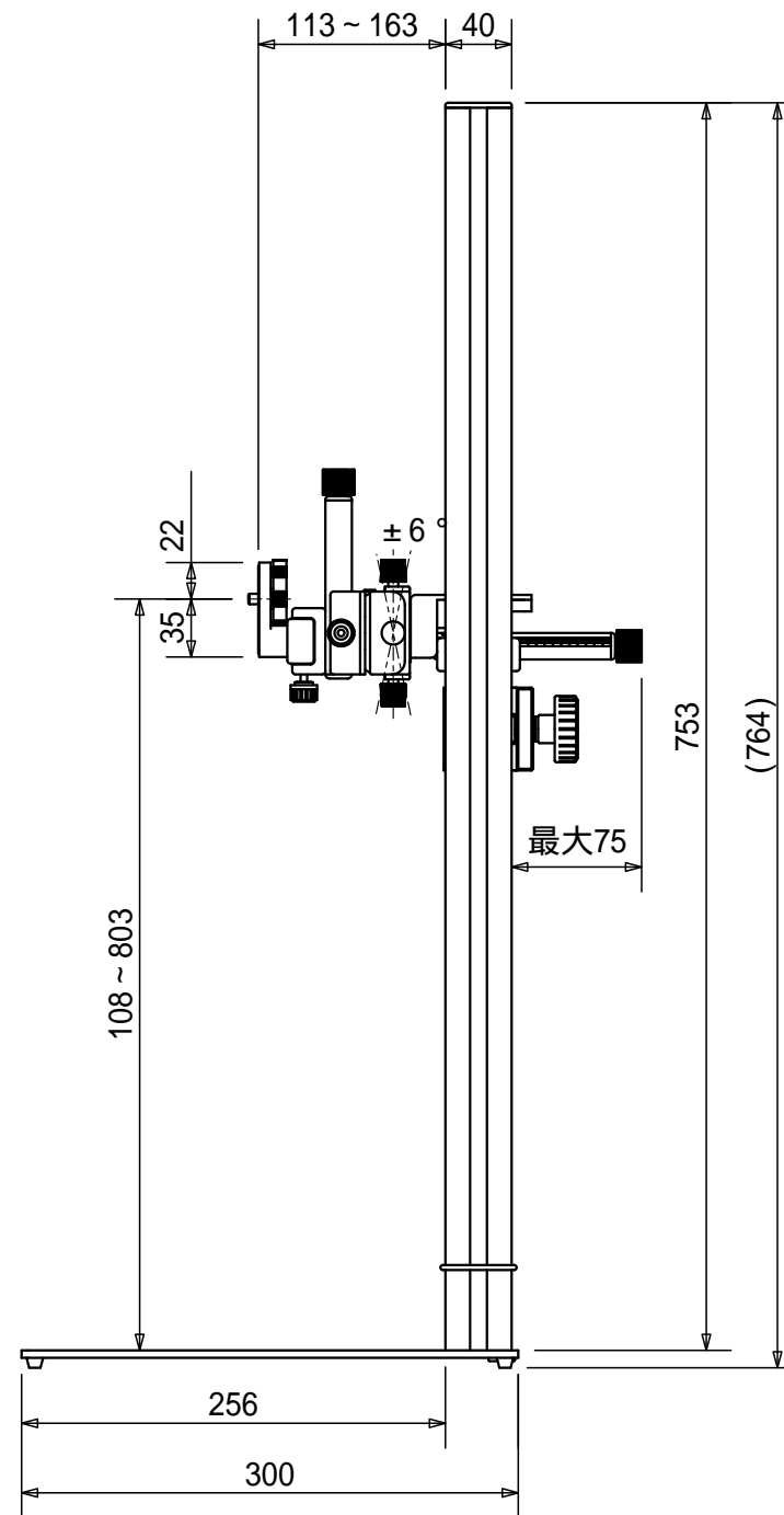
カメラスタンドMK - XYZL(750)
