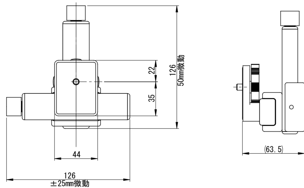
詳細図 カメラ取付部 尺度1:1
