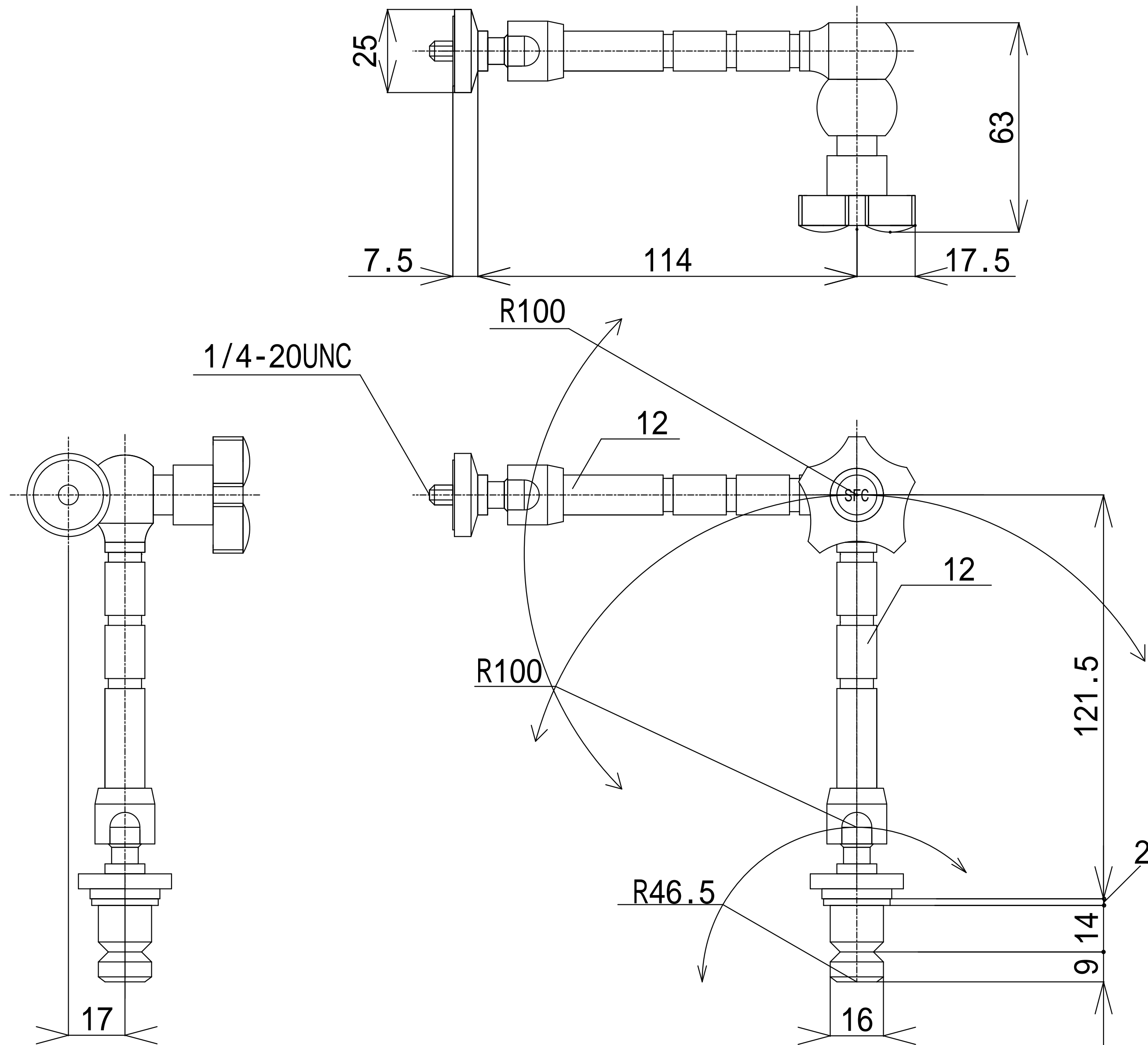
フレキシブルアーム(本体)ロングタイプ
