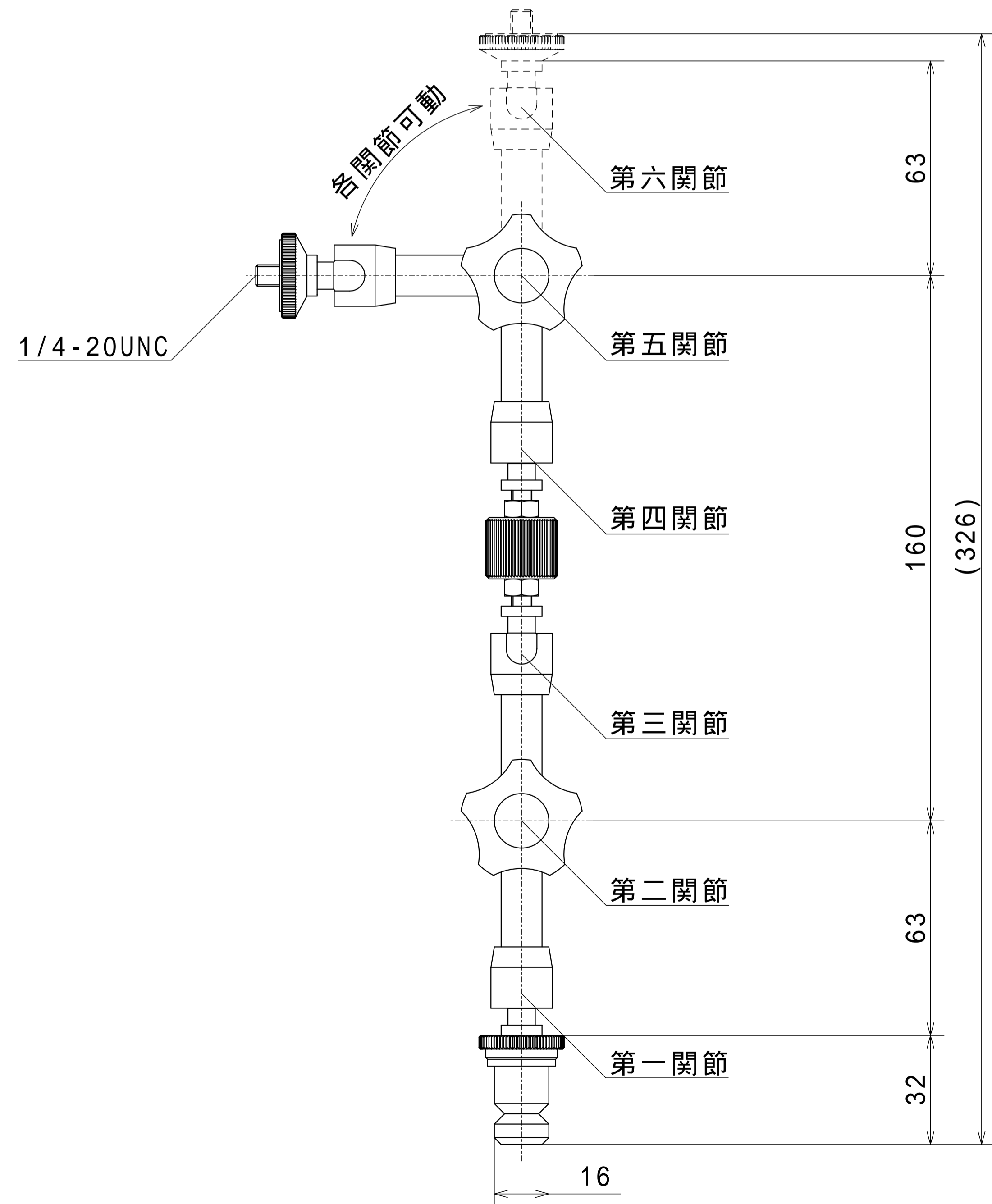
フレキシブルアーム(本体)ダブルジョイント
