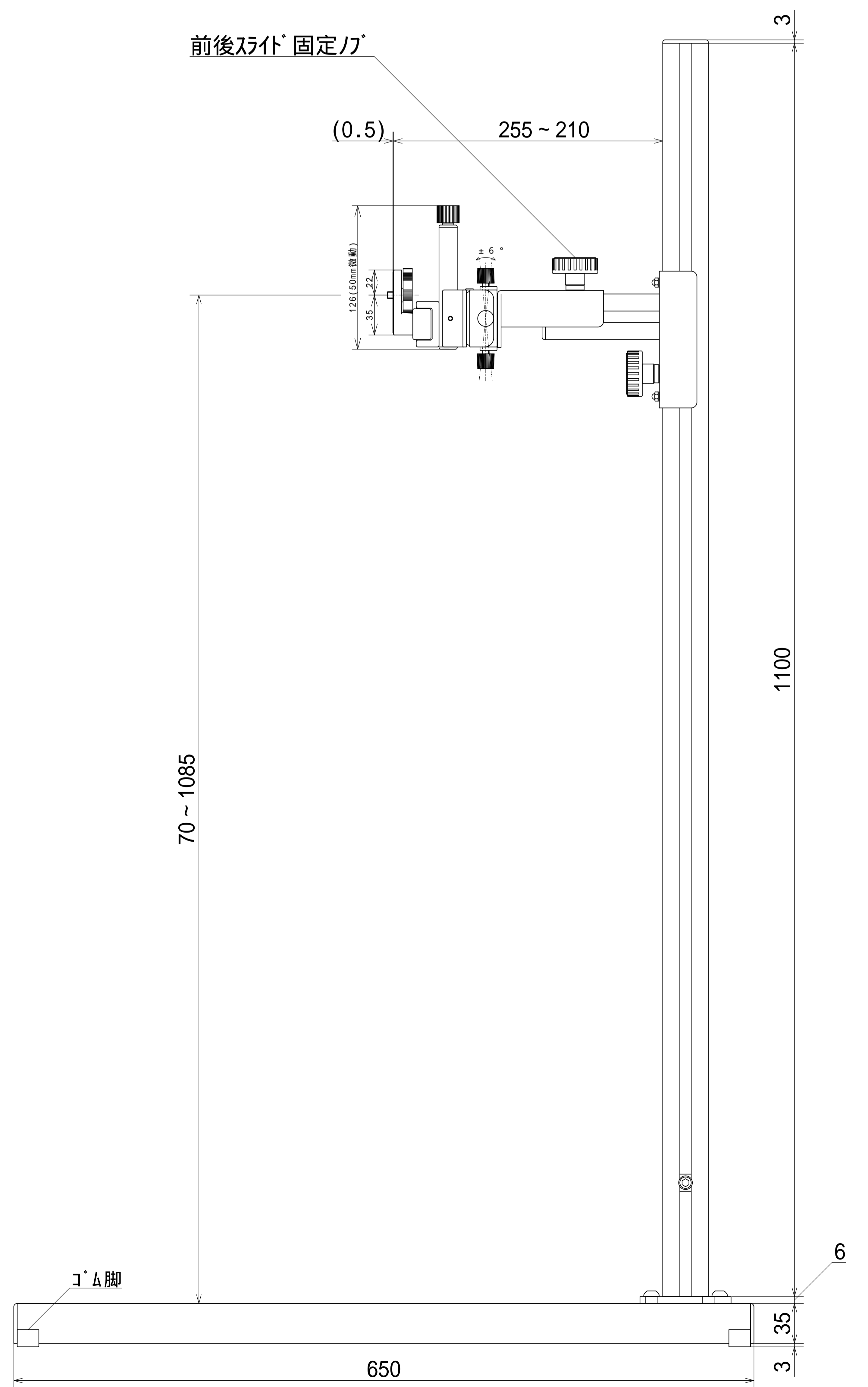
カメラスタンド1100XY-L
