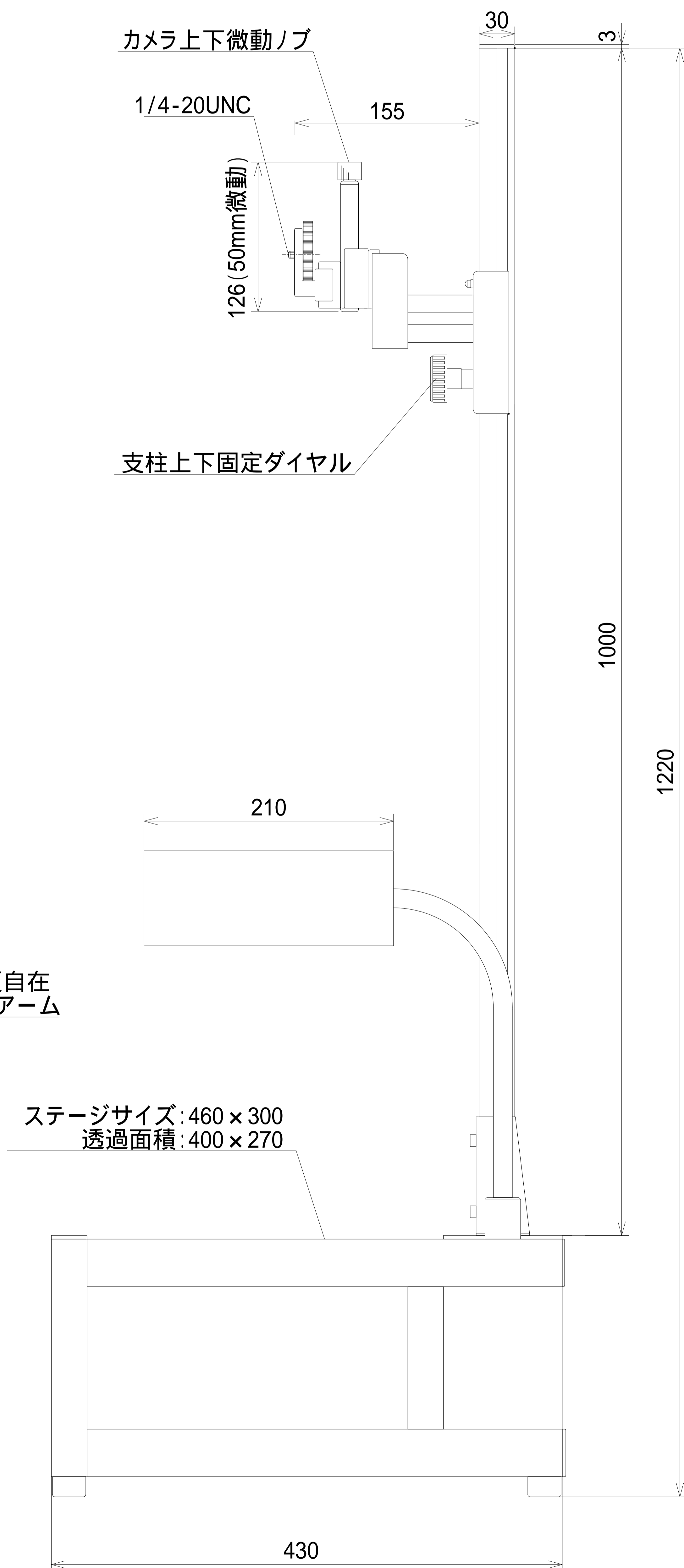
カメラスタンドC-DL-LED
