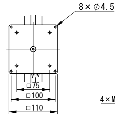
詳細図 B
