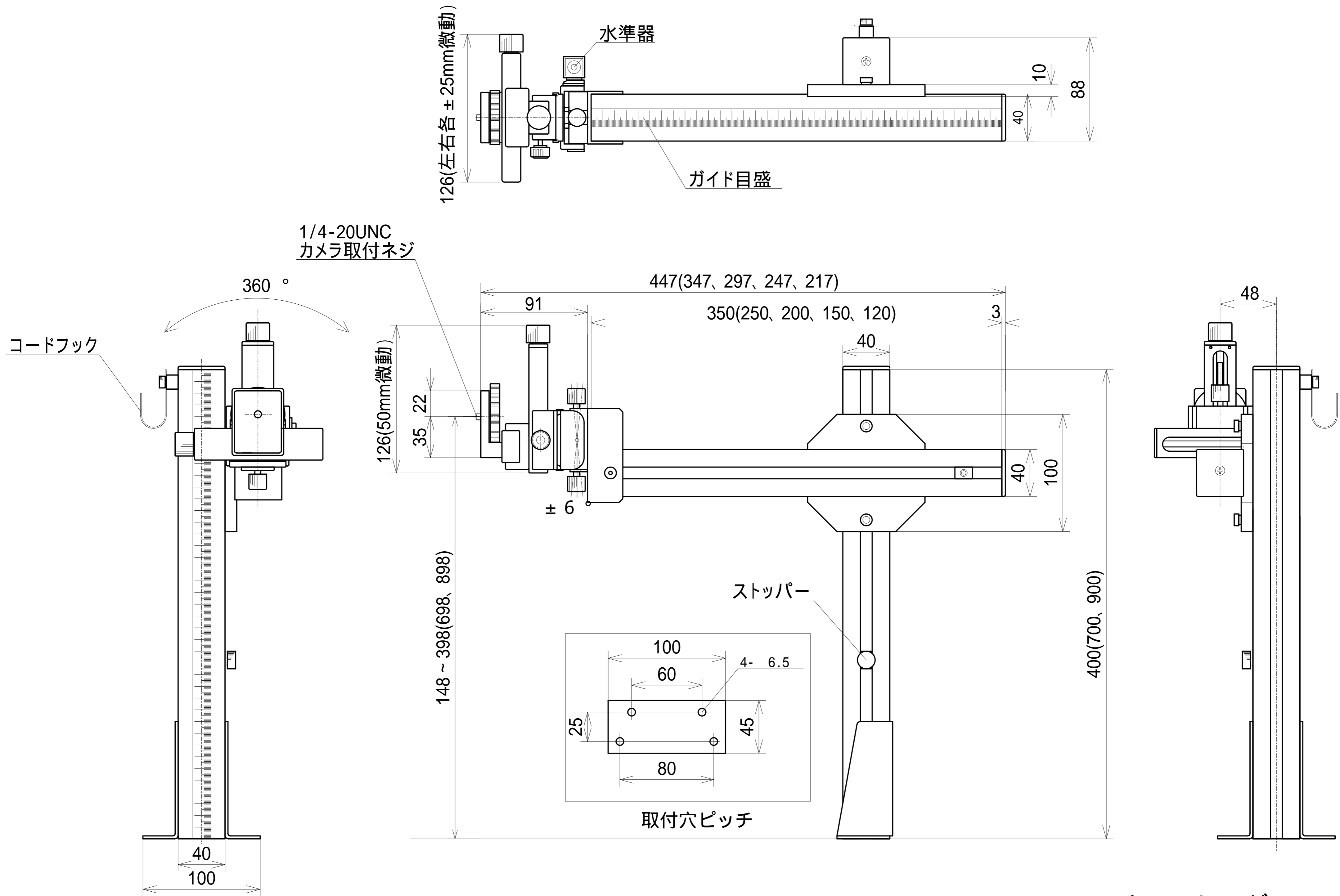
マルチカメラホルダー-S
