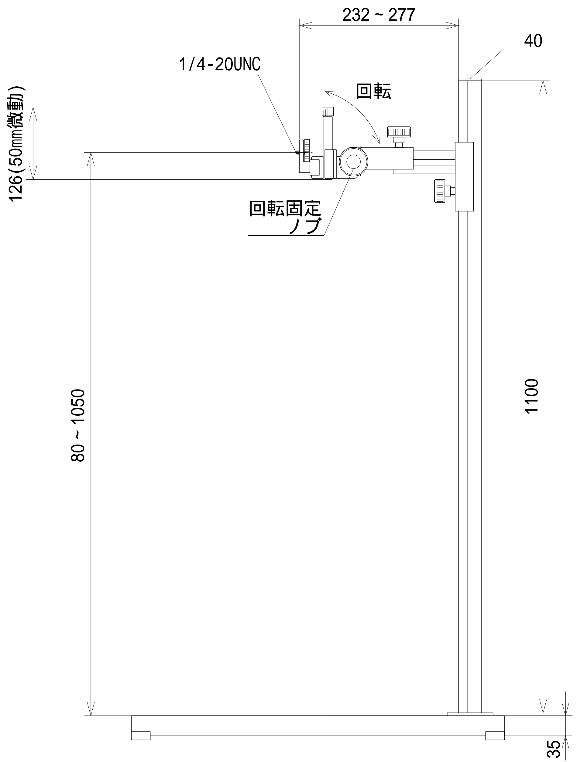
カメラスタンド1100-VH
