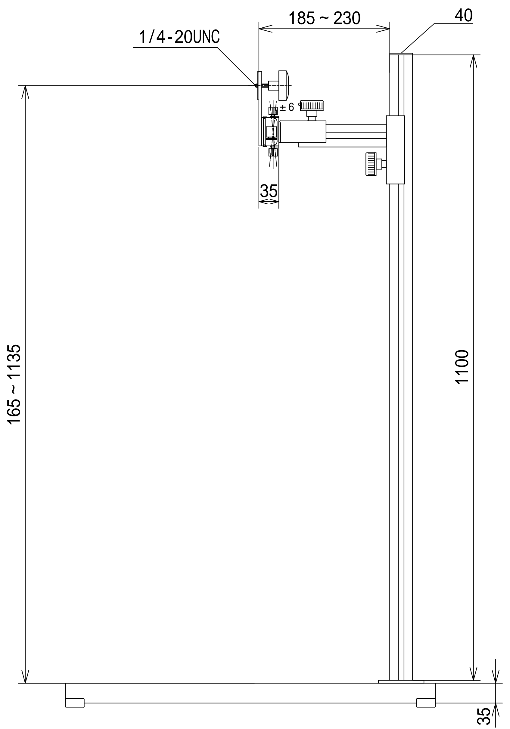
カメラスタンド1100 - PL
